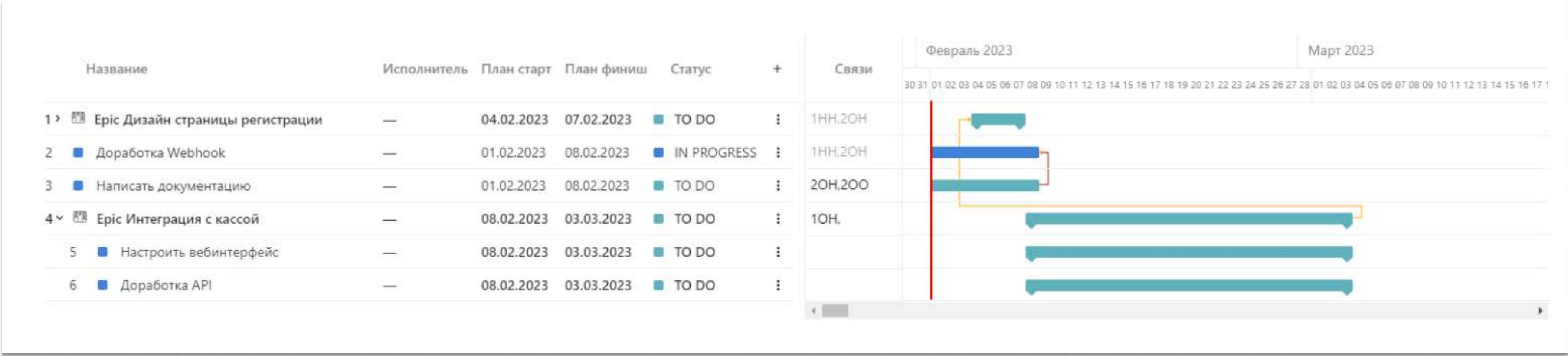
Диаграмма Ганта
